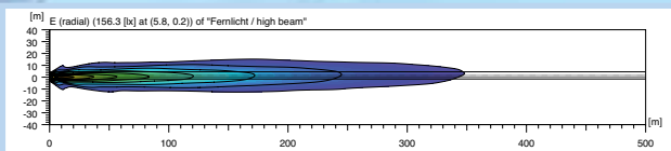
Vergelijkbare schijnwerper zonder High-Boost-reflector
